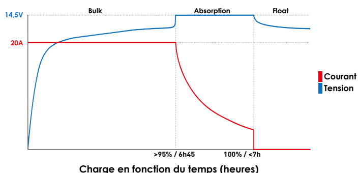
Profil de charge à courant et tension constants (CC/CV) recommandé
